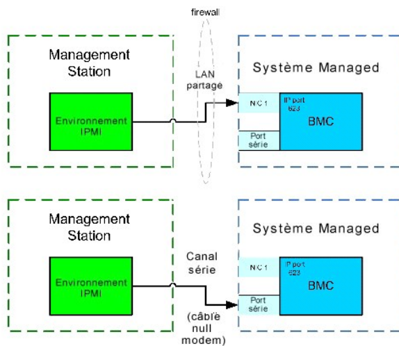
Figure 3-2. Schéma de l'environnement IPMI
